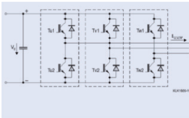
Topología de 2 niveles Convencional (6 IGBT)
