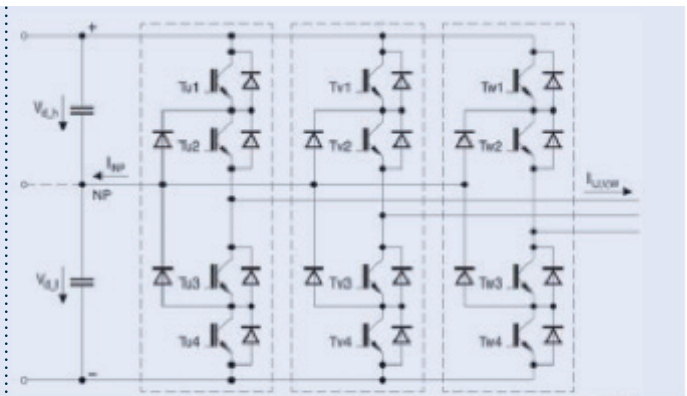
Topología de 3 niveles smARTline™ (12 IGBT)
